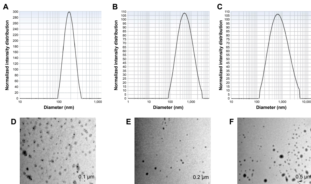
Figure 2 DLS measurement, nanoparticle size measurement of (A) PLGANP, (B) PLGA -GF NP, and (C) PLGA -GF -K4 NP and TEM images of (D) PLGANP, (E) PLGA -GF NP, and (F) PLGA -GF -K4 NP.
